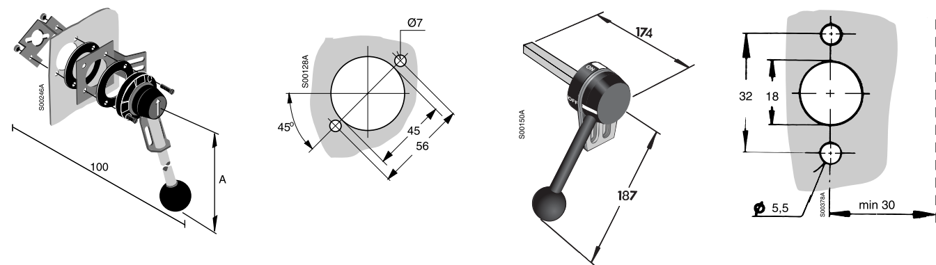
Отверстие в дверце под ручку управления YASDA
