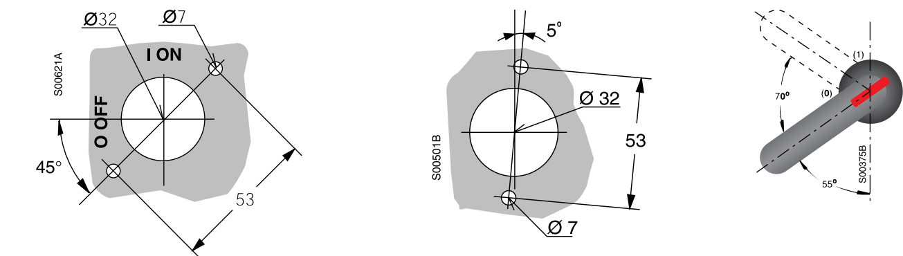
Отверстие в дверце под ручку управления ОН_
