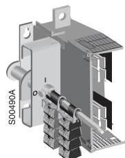
Максимум 8+8 доп. контактов OZXK 1...6 (выключатели 630...800A)
